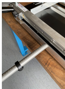
Maßskala + Bajonetteverschluss auf beiden Längenanschlagsrohren Measure Scale + Bayonet lock on both length stop tubes
